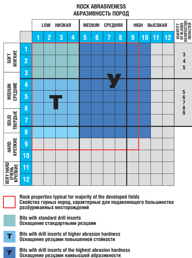
● Fig. 1 Range of application of BURINTEKH drill bits ● Рис. 1 Область применения долот производства ООО НПП «Буринтех»
